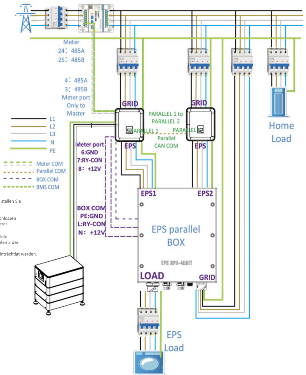
Systemdiagramm von zwei H3 offline und parallel
